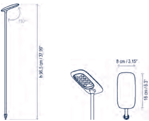
Birdie Luminaria 100L / Birdie Luminaire 100L
