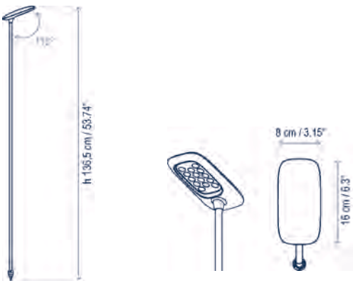
Birdie Luminaria 140L / Birdie Luminaire 140L
